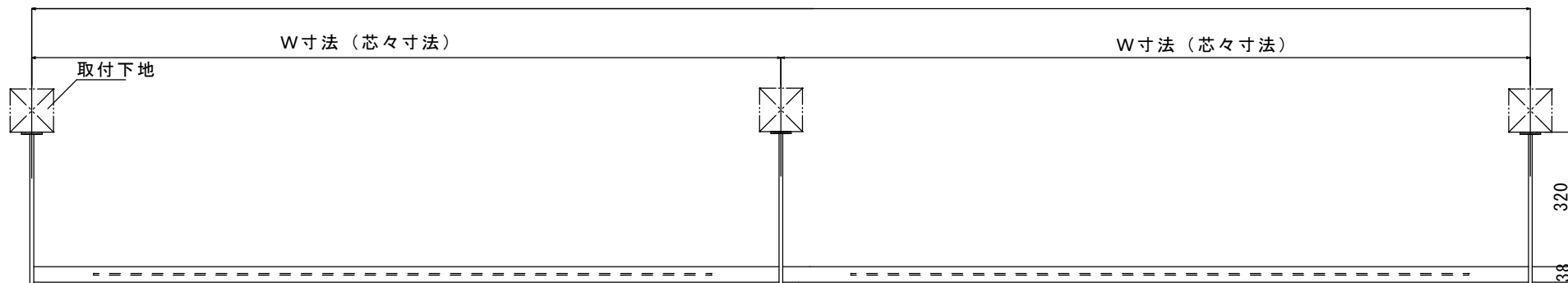
W寸法 (芯々寸法)
