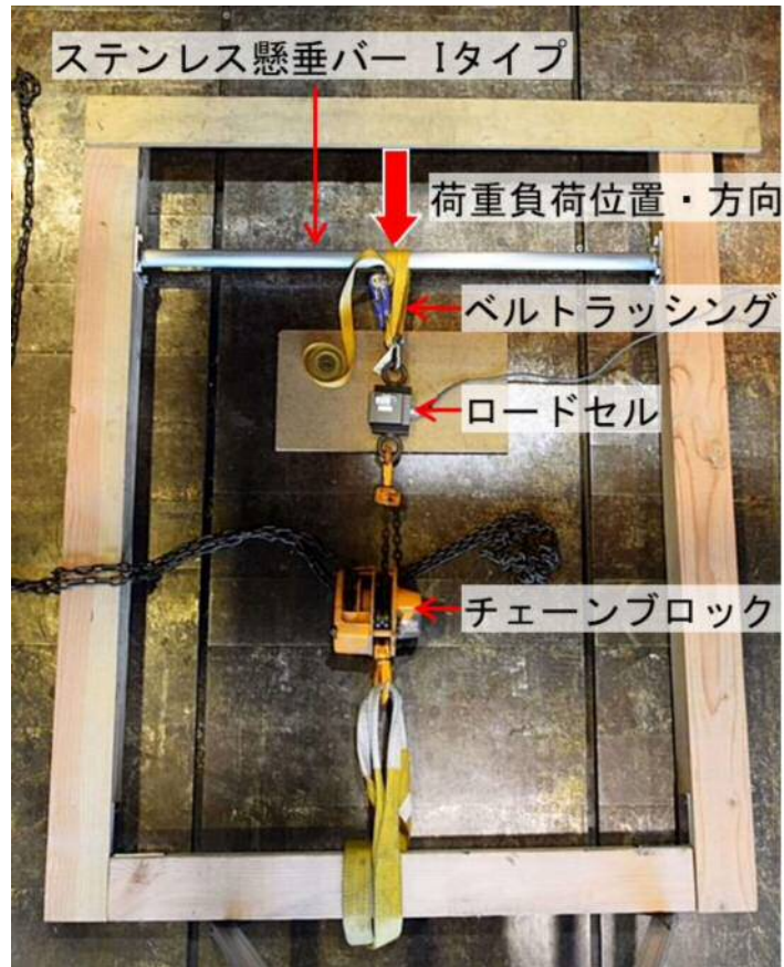
図1 試験1の耐荷重試験状況
