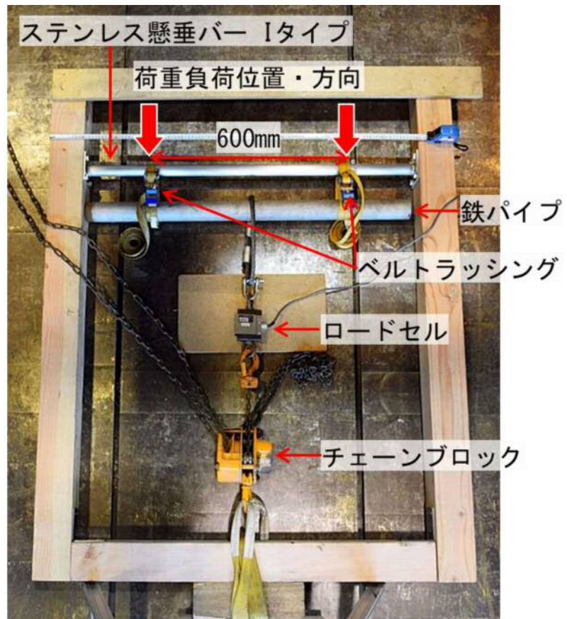
図2 試験2の耐荷重試験状況
