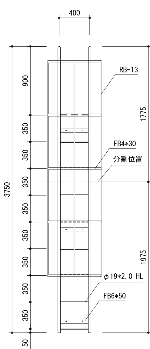
姿図
