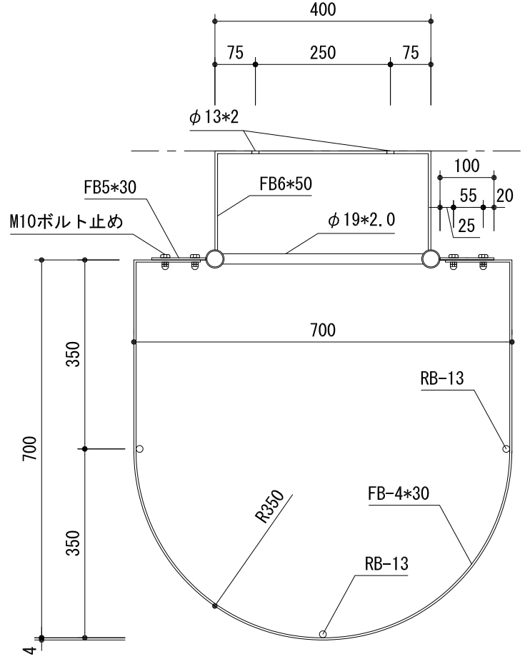
平面詳細図
